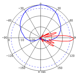
1710-2490MHz: \pm 45^\circ Pol.
