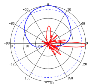
2490-2690MHz: \pm 45^\circ Pol.
